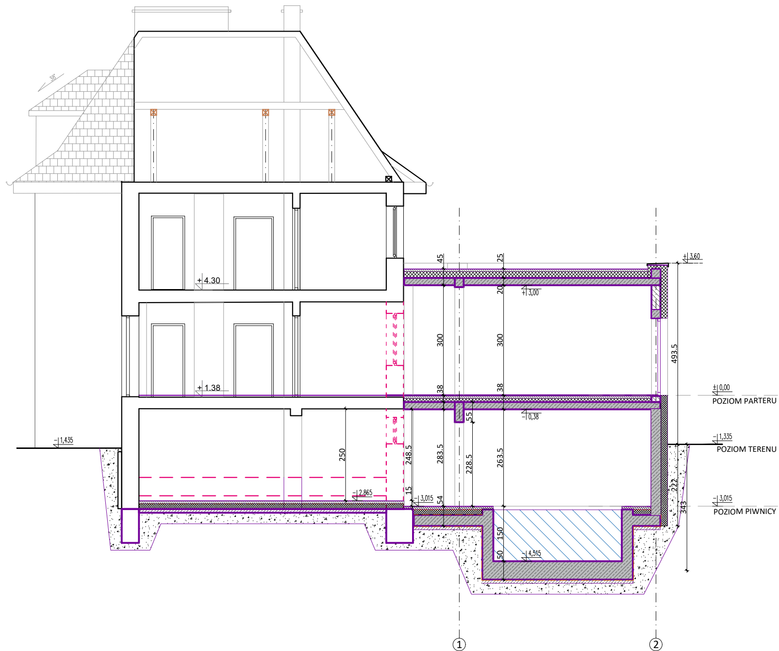
PRZEKRÓJ AA
